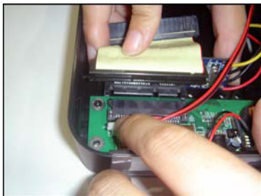
3. Если вы хотите использовать диск PATA подключите его через переходник
