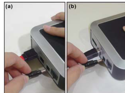
11a. После подключения eSATA кабеля к внешнему накопителю, подключите к накопителю кабель питания. 11b. После подключения USB кабеля к внешнему накопителю, подключите к накопителю кабель питания.
